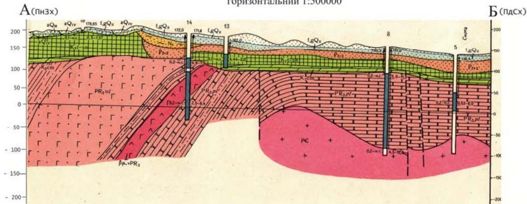
Гідрогеологічний розріз по лінії А-Б Масштаб: вертикальний 1:5000 горизонтальний 1:500000
